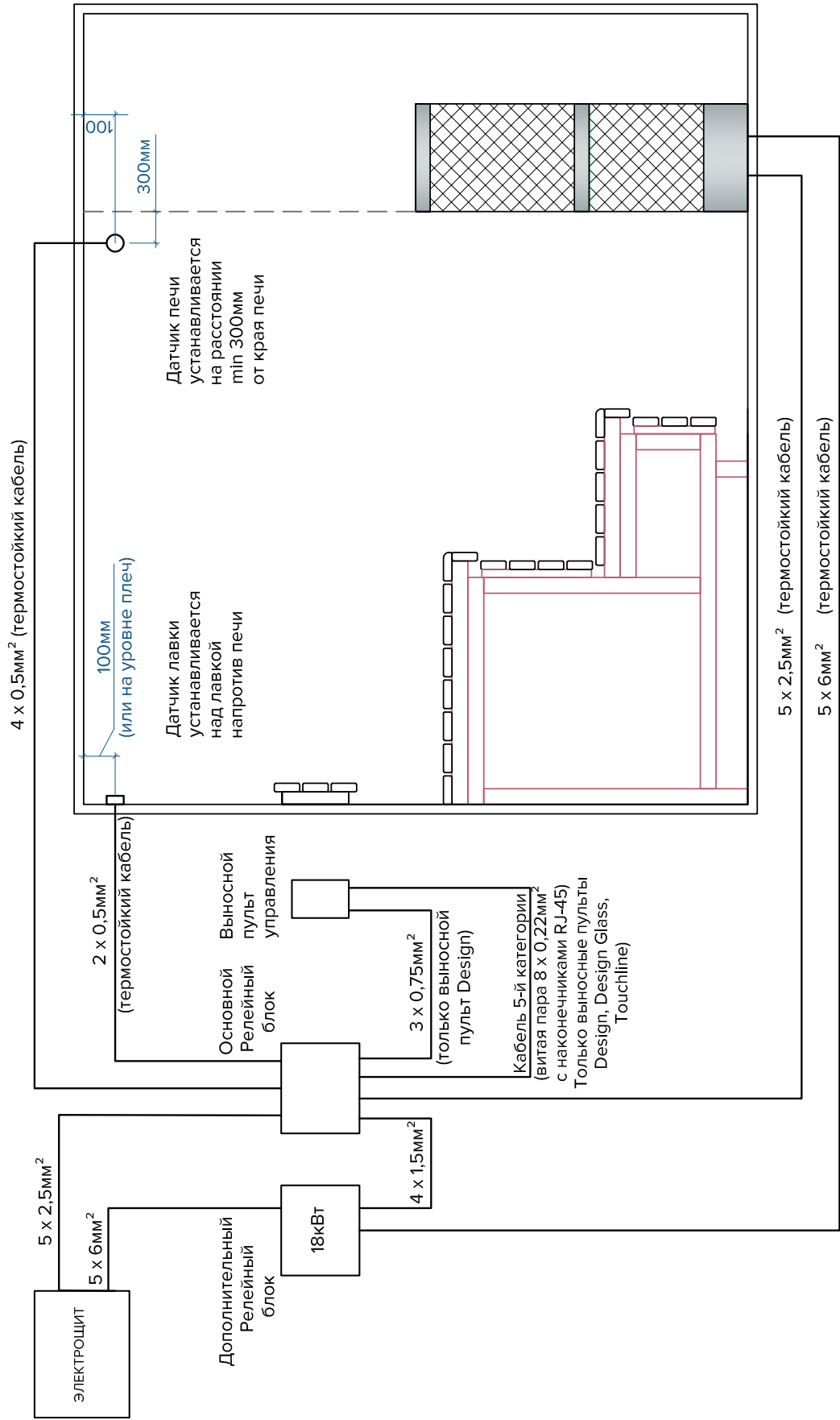
Схема установки печей IKI Pillar 20кВт (5+15 кВт) + панель управления Fasel
